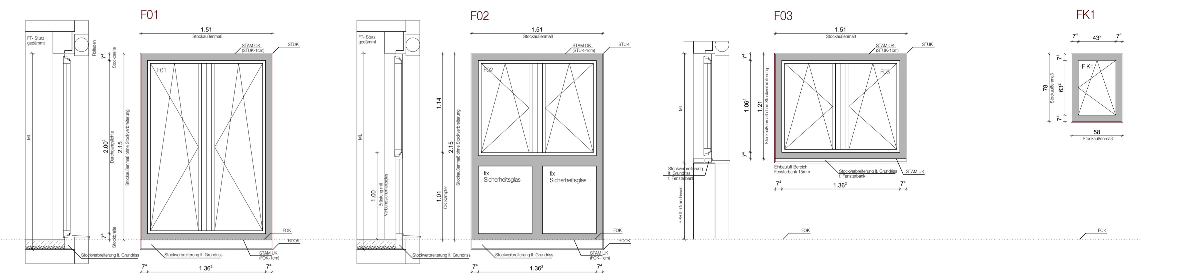
FENSTERTYPEN M 1:25
